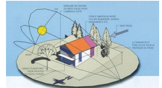
Principes de construction bioclimatiques
