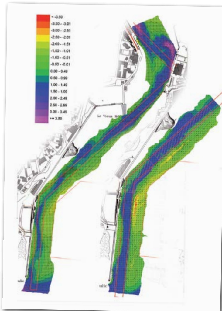
Relevés bathymétriques avant et après dragages
