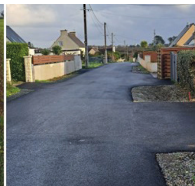
Réfection de chaussée, gestion pluviale et limitation de vitesse – Rues Ar Goarem (Pont-Croix) & Matelot Pochic
